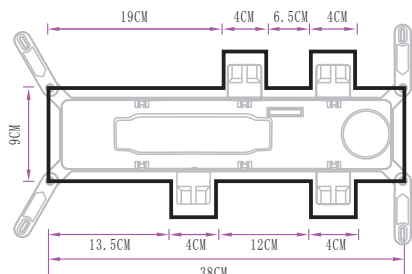
阀体开槽尺寸
